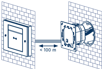
Abgesetzte Montage
