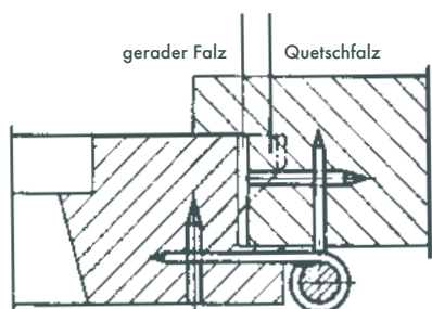
Rahmenlappen auf Mitte für geraden und Quetschfalz
